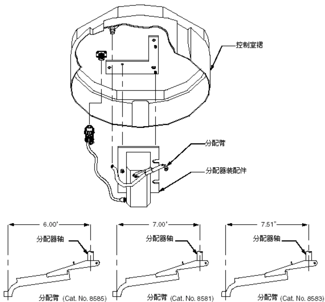
图16 分配器安装
