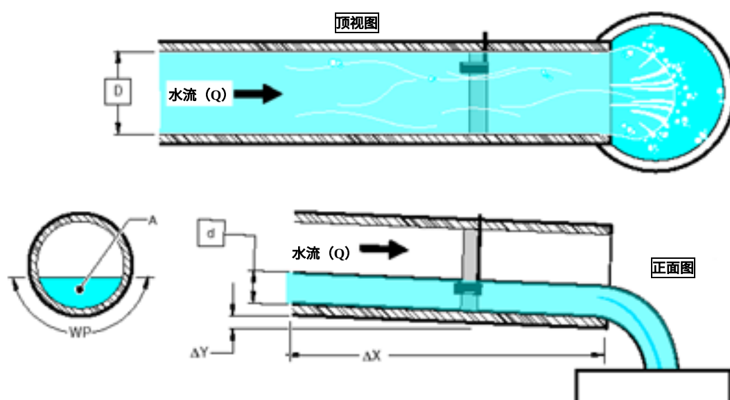
图 55 圆形管道
