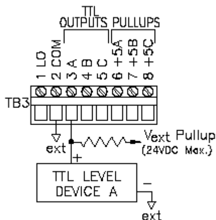
图 2-8 外部供电逻辑操作的 TTL 输出连接
