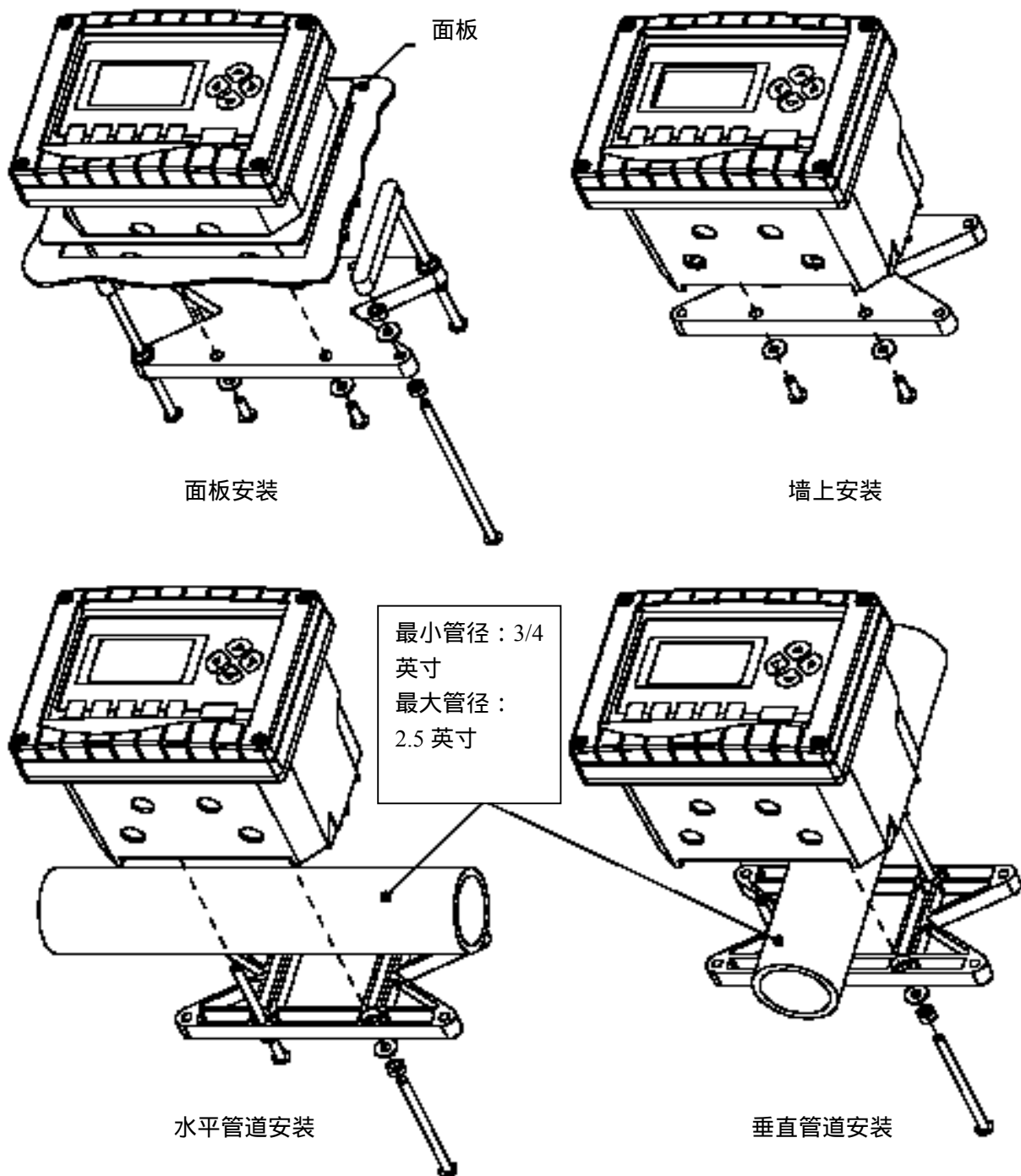
图 2-1 测定仪安装型式
