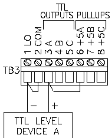
图 2-7 内部供电逻辑操作的 TTL 输出连接
