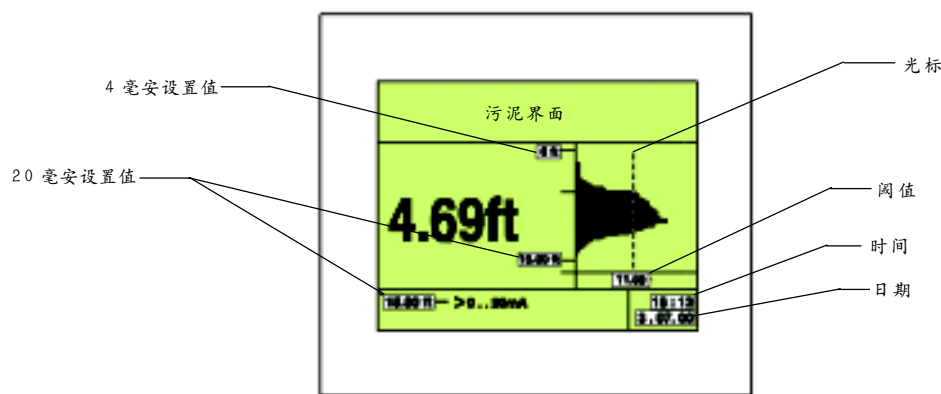
图6 图形测量模式显示（图形显示）
